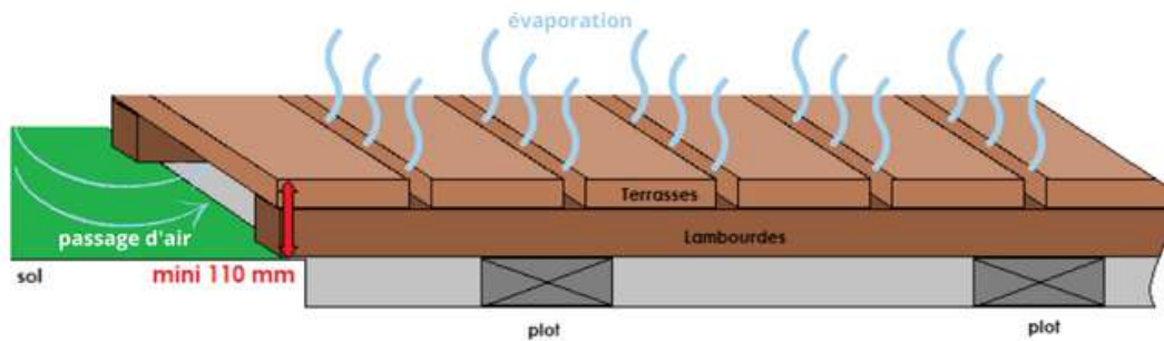
Illustration de l'importance de la ventilation latérale préconisée par le DTU 51-4 sur les bois en classe emploi 3.
